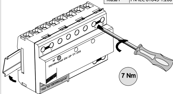
Rys. 1 Układ sieci TT układ 1+1 - Podłączenie
