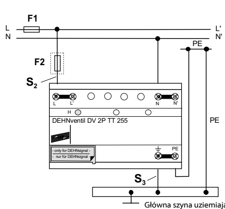
Rys. 2 Układ sieci TT układ 1+1 - Podłączenie
