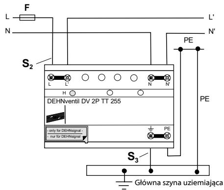
Rys. 2 Układ sieci TT układ 1+1 - Podłączenie
