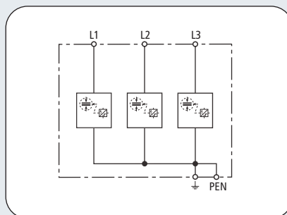
Schemat połączeń DSH TNC 255
