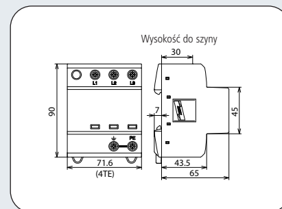
Rysunek wymiarowy DSH TNC 255
