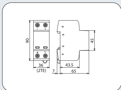
Rysunek wymiarowy DSH TN 255
