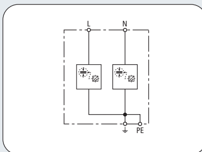
Schemat połączeń DSH TN 255
