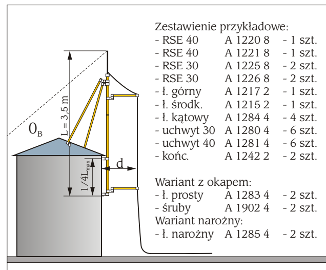
Rysunek 18. Ochrona metalowego obiektu zwodem odsuniętym.
