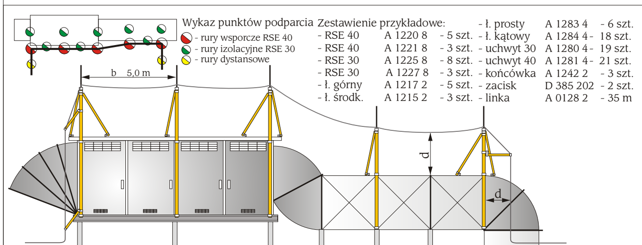
Rysunek 19. Ochrona centrali wentylacyjnej zwodami odsuniętymi systemu AntyGrom. W rozwiązaniu założono możliwość nitowania łączników kątownych do obudowy. Przy dokładnej znajomości detali centrali można zaprojektować mocowanie rur za pomocą kłm felcowych - bez konieczności dziurawienia obudowy!!!
