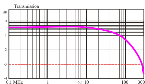
Typowe charakterystyki tłumienia i fali odbitej.
