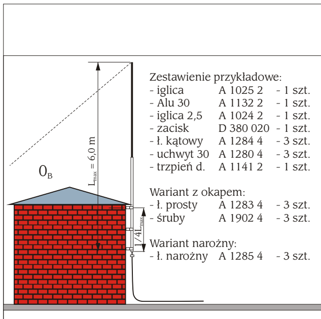
Rysunek 17. Ochrona nie metalowego obiektu aluminiowym zwodem pionowym.
