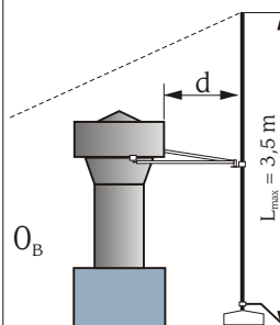
Rysunek 12. Ochrona wentylatora iglicą odgromową wspartą drążkami izolacyjnymi na jego obudowie.
