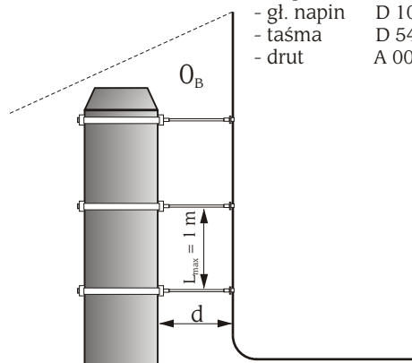
Rysunek 13. Ochrona komina pieca c.o. ze stali nierdzewnej zwodem z drutu odgromowego.
