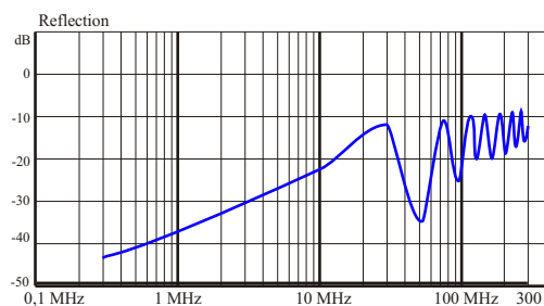
Typowe charakterystyki tłumienia i fali odbitej.
