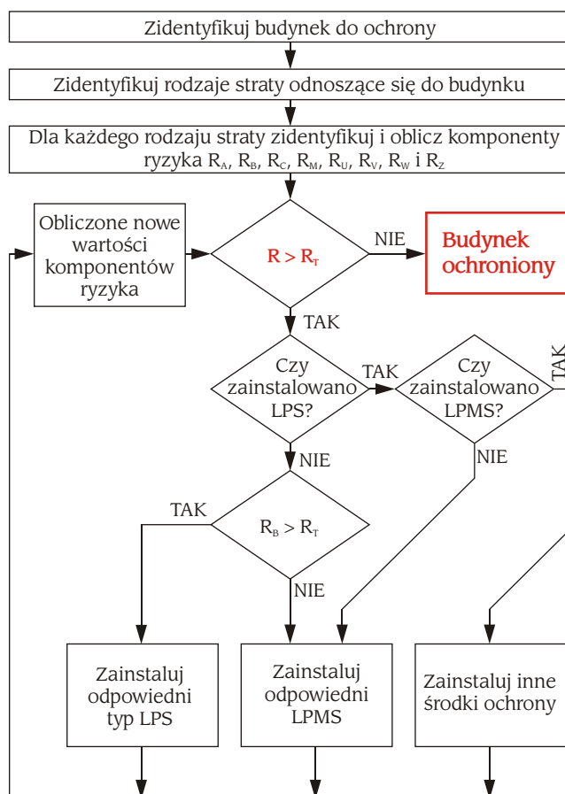
Rysunek 1. Procedura wyboru środków ochrony w budynku.
