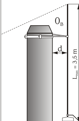
Rysunek 14. Ochrona komina ze stali nierdzewnej iglicą opartą na drążkach izolacyjnych.
