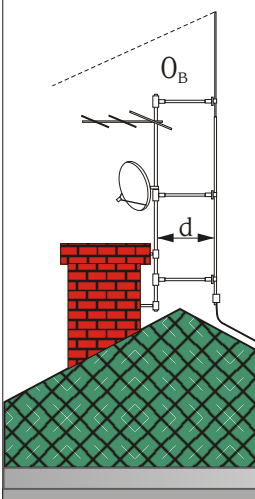
Rysunek 16. Ochrona zespołu anten RTV+SAT iglicą odgromową zamocowaną na wspornikach izolacyjnych serii A 1310 8.
