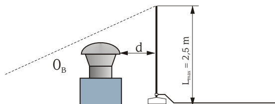
Rysunek 11. Ochrona niewielkiego wentylatora iglicą odgromową wolnostojącą.
