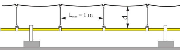
Rysunek 15. Ochrona rury gazowej zwodem z linki odgromowej A 0128 2.
